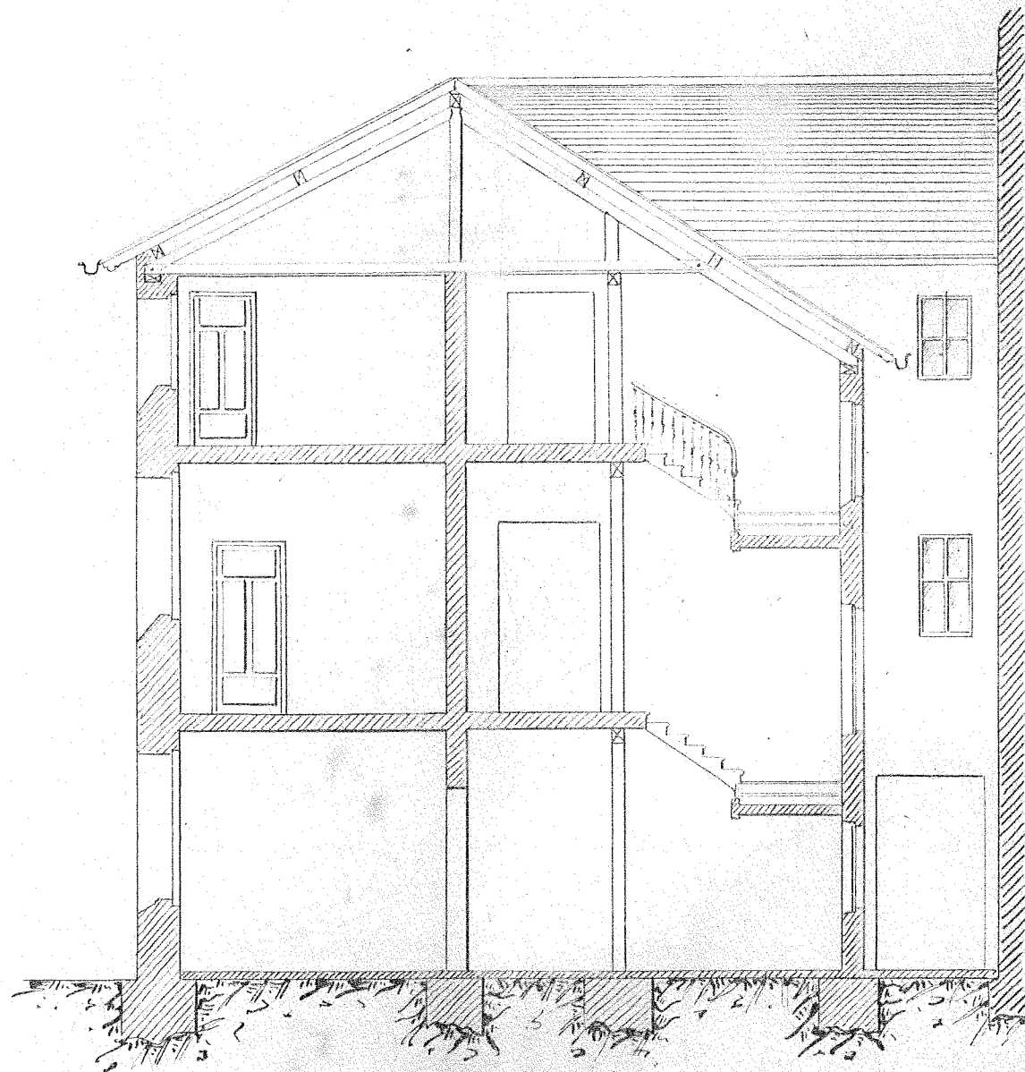
SECCION POR A.B.
