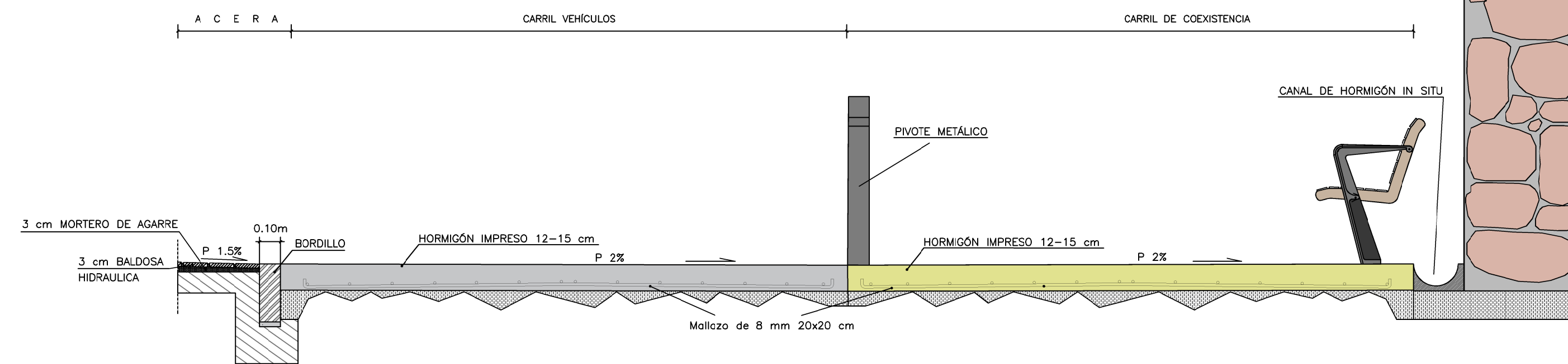
DETALLE B-B'
