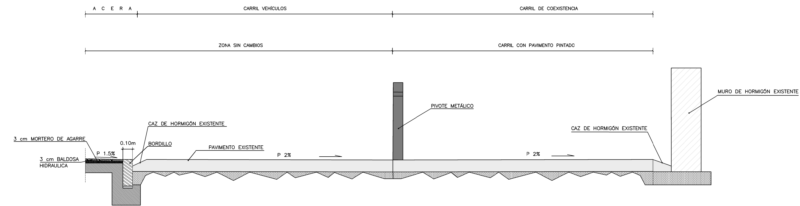
DETALLE C-C'
